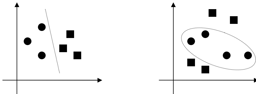
شکل (3-2) : بعد VC
